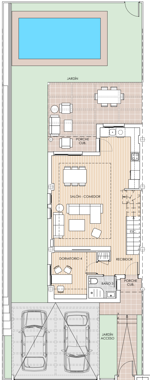
PLANTA BAJA
