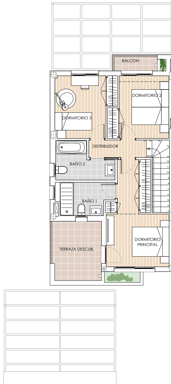
PLANTA PRIMERA
