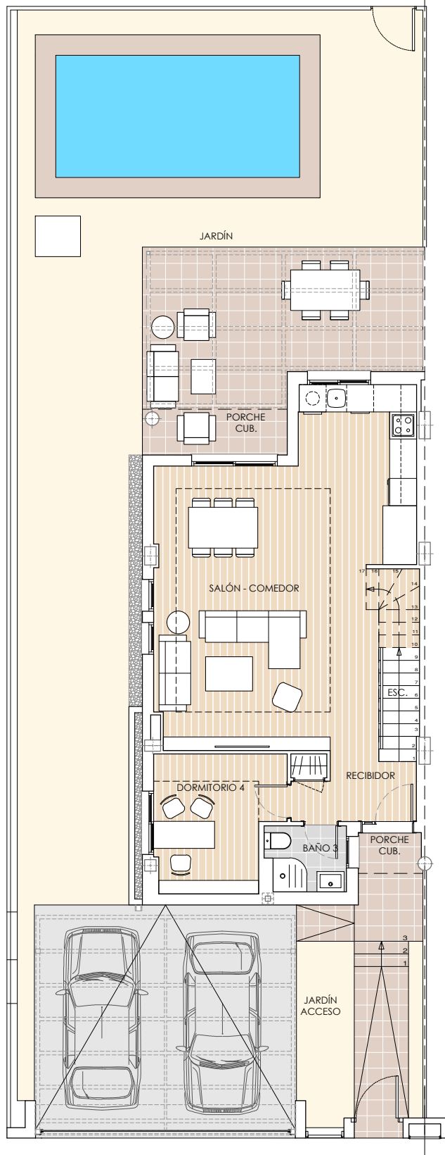
PLANTA BAJA
